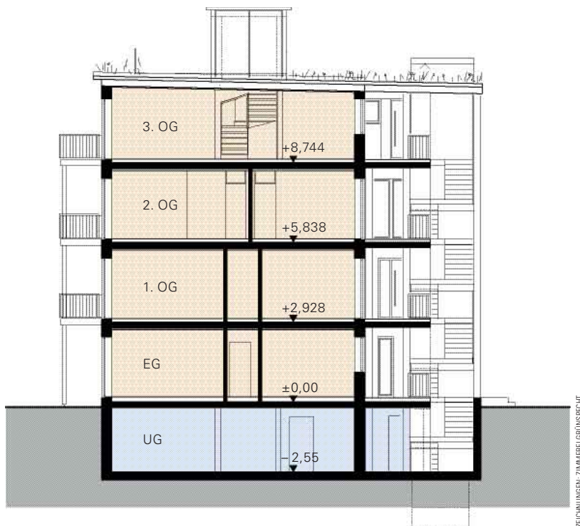
Querschnitt A-A
